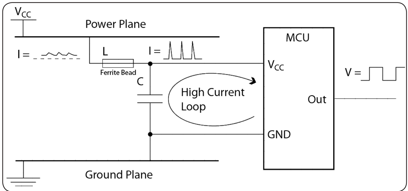
شکل (۲): مکان قرار گرفتن بهتر خازن‌های دکوپلینگ
