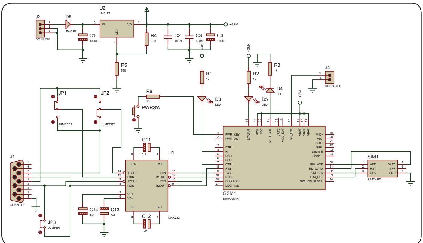
مدار کلی یک GSM مودم نمونه با استفاده از ماژول Sim900 و ارتباط از طریق درگاه سریال رایانه
