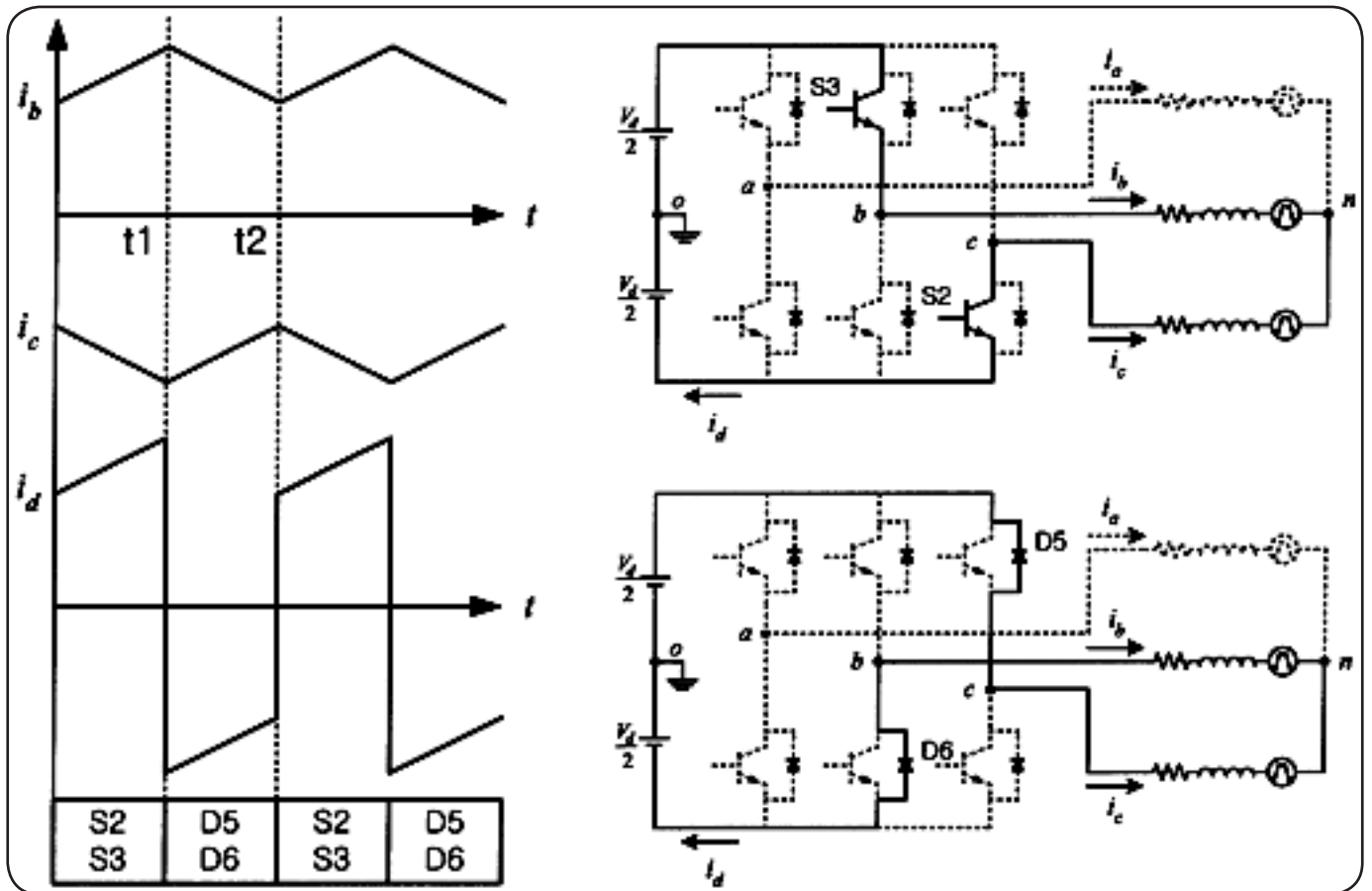
شکل ۳ عملکرد مد نرمال
