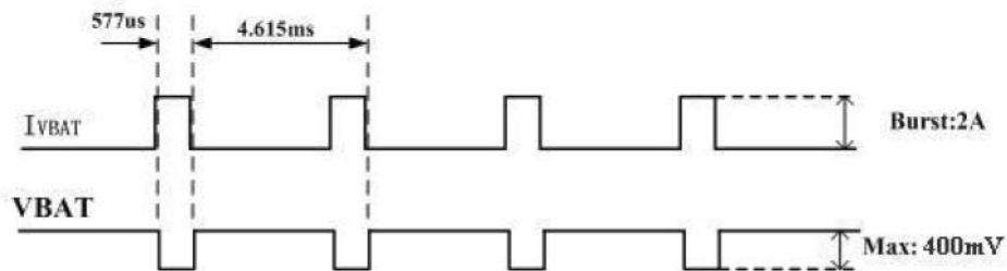
شکل موج جریان ماژول SIM900
