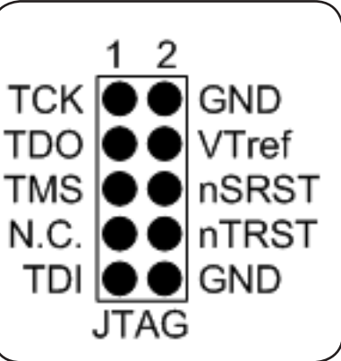
شکل (۷): کانکتور JTAG استاندارد
