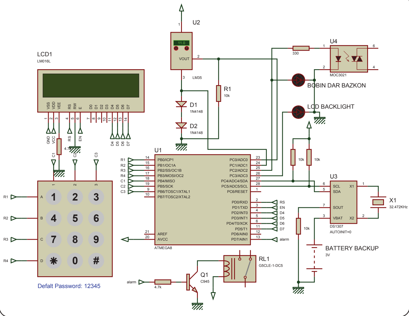
شکل ۱: شماتیک مدار
