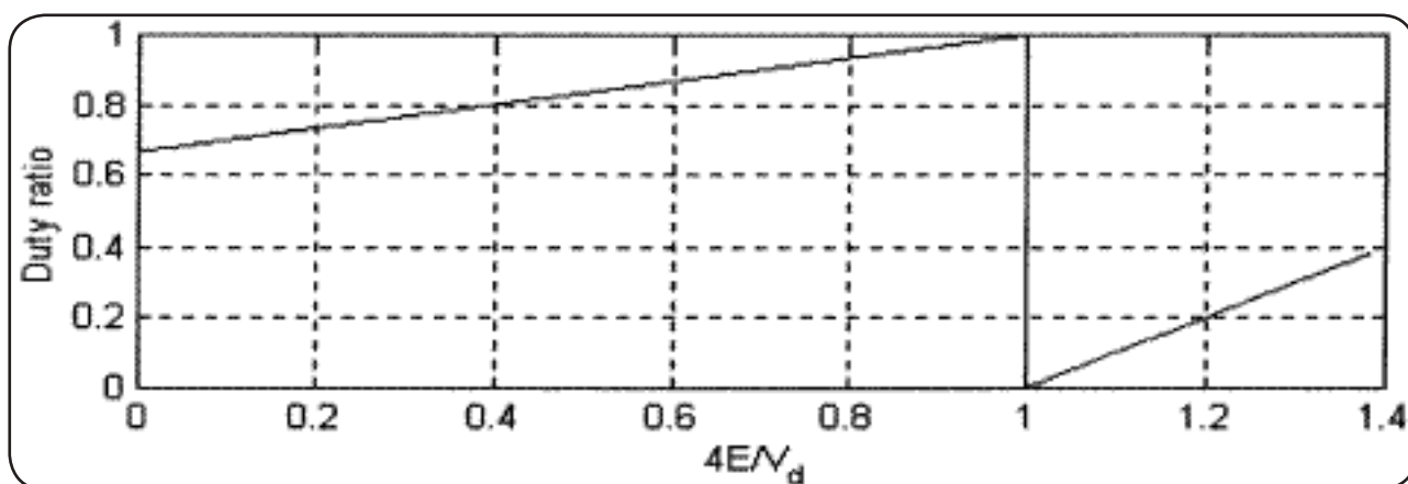
شکل ۷ نسبت D برای جبران سازی کموتاسیون
